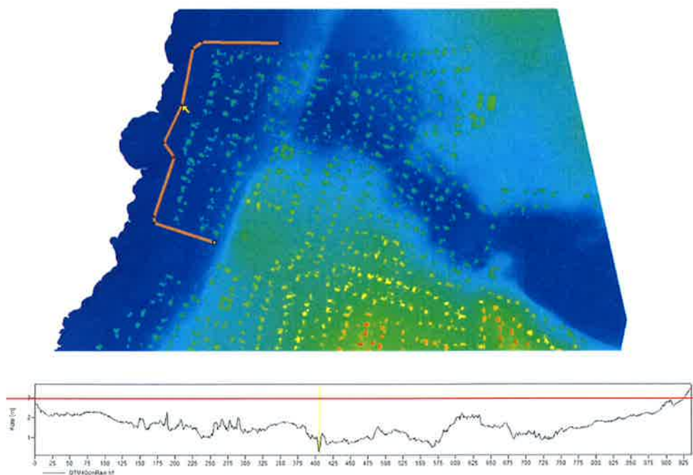
Figur 21 Over Dråby Strand Nord. Længdesnit af det eksisterende terræn langs diget. Den røde linje markerer den fremtidige digehøjde.
