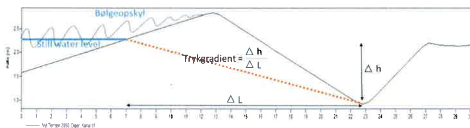
Figur 11 Skitse til bestemmelse af trykgradient
