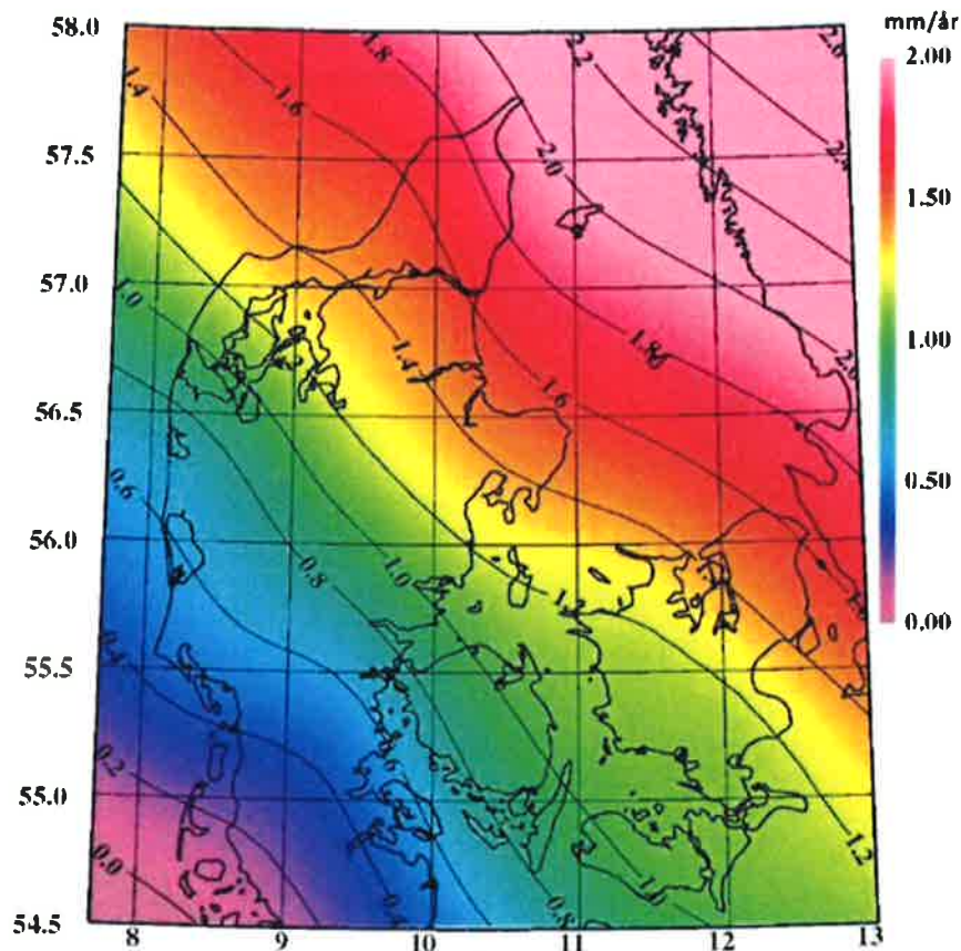
Figur 8 Absolutte rater for landhævning i Danmark. Kilde: /4/
