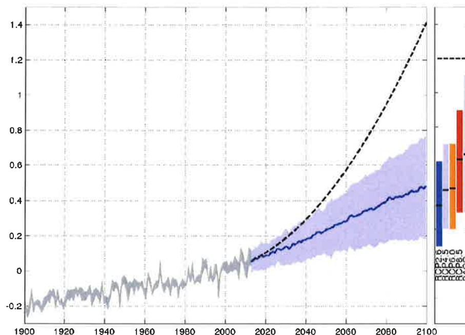
Figur 6 Den absolutte middelvandstand ved Danmark i meter for årene 1900-2100. Den grå skygge for år 1900-2012 viser den observerede årlige middelvandstand ved danske vandstandsmålere, korregeret for landhævning. Den blå streg for år 2012-2100 viser IPCC's bedste estimat af middelvandstanden i Nordsøen for RCP4.5 scenariet, og skyggen angiver usikkerheden for dette scenarie. Den stiplede linje angiver DMI's estimat af en øvre grænse for vandstandsstigninger til brug for usikkerhedsberegninger. I højre side af figuren vises middelværdi og usikkerheder for de fire IPCC scenarier samt for BACC's vurdering af A1B scenariet for perioden 2081-2100. Den stiplede linje viser DMI's øvre bud for denne periode. Kilde: /3/.
